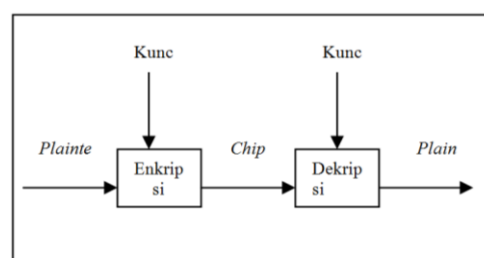
Gambar 1 Kriptografi Simetri
